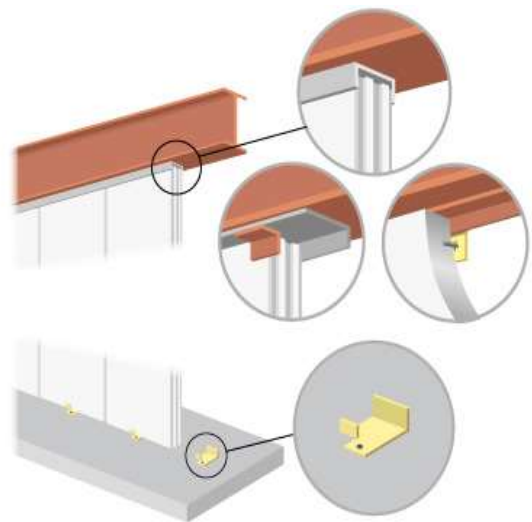
縦壁フットプレート構法
