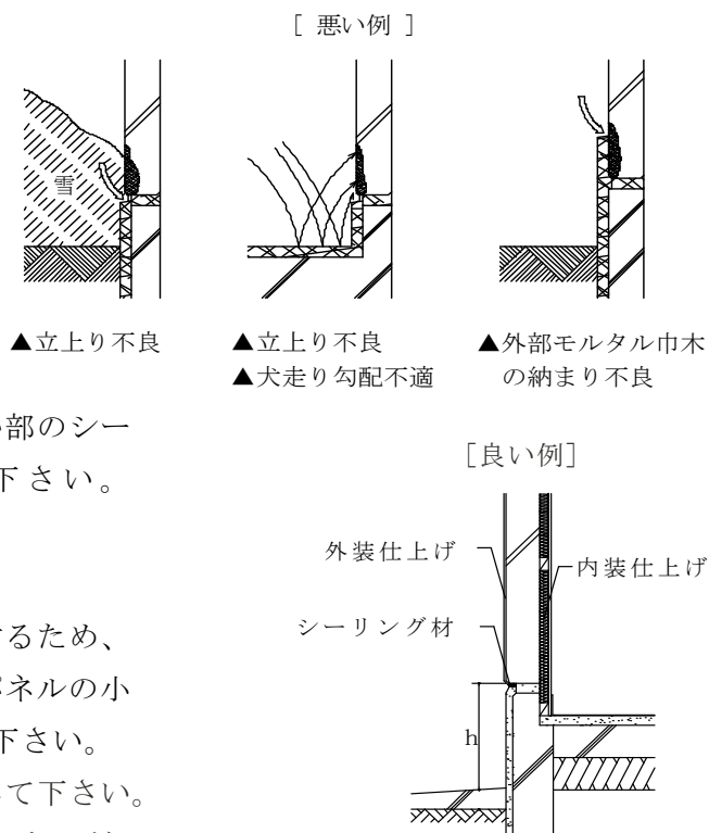
図-15 布基礎の例
